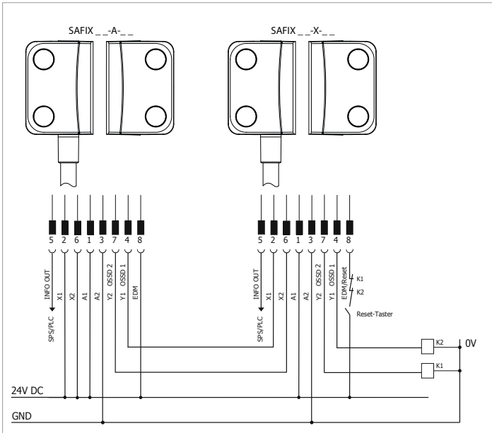
Abb. 10: Direkter Anschluss zweier Schützen nach PL e, SAFIX __-A-__ & SAFIX __-X-__ Der Eingang EDM wartet auf eine Startpulsdauer zwischen 30 ms und 5 s. Am EDM Eingang sind ebenfalls die Rückführkreise der Schütze K1 und K2 angeschlossen.
