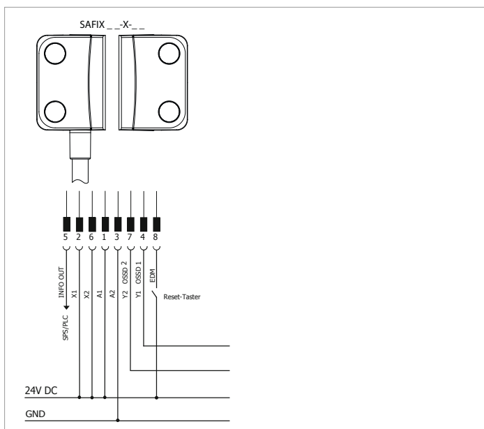
Abb. 7: Eingang eines Reset-Tasters Für die Variante EMD-Eingang überwacht (SAFIX __-X-__) Die Eingänge X1 und X2 werden mit 24 V DC beschaltet. Die Ausgänge Y1 und Y2 werden auf die Auswertung geführt. Der Diagnoseausgang kann z.B. an eine SPS angeschlossen werden. Der Eingang EDM wartet auf eine Startpulsdauer zwischen 30 ms und 5 s.
