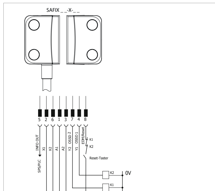
Abb. 9: Direkter Anschluss zweier Schützen nach PL e, SAFIX __-X-__ Die Eingänge X1 und X2 werden mit 24 V DC beschaltet. Die Ausgänge Y1 und Y2 werden auf die Auswertung geführt. Der Diagnoseausgang kann z.B. an eine SPS angeschlossen werden. Der Eingang EDM wartet auf eine Startpulsdauer zwischen 30 ms und 5 s. Am EDM Eingang sind ebenfalls die Rückführkreise der Schütze K1 und K2 angeschlossen.
