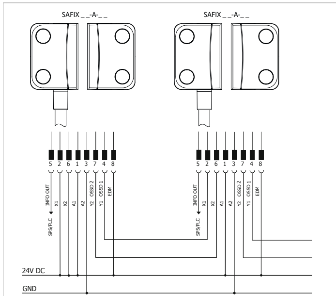
Abb. 6: Reihenschaltung mit Diagnoseausgang, automatischer Reset Für die Variante EMD-Eingang automatisch (SAFIX __-A-__) Die Eingänge X1 und X2 werden mit 24 V DC beschaltet. Die Ausgänge Y1 und Y2 werden auf die Auswertung geführt. Der Diagnoseausgang kann z.B. an eine SPS angeschlossen werden.
