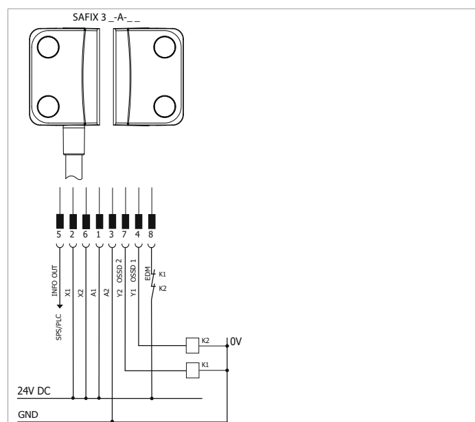
Abb. 5: Anschluss mit Diagnoseausgang, automatischer Reset
