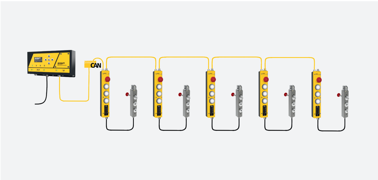
*Darstellung CAN-Vernetzung
