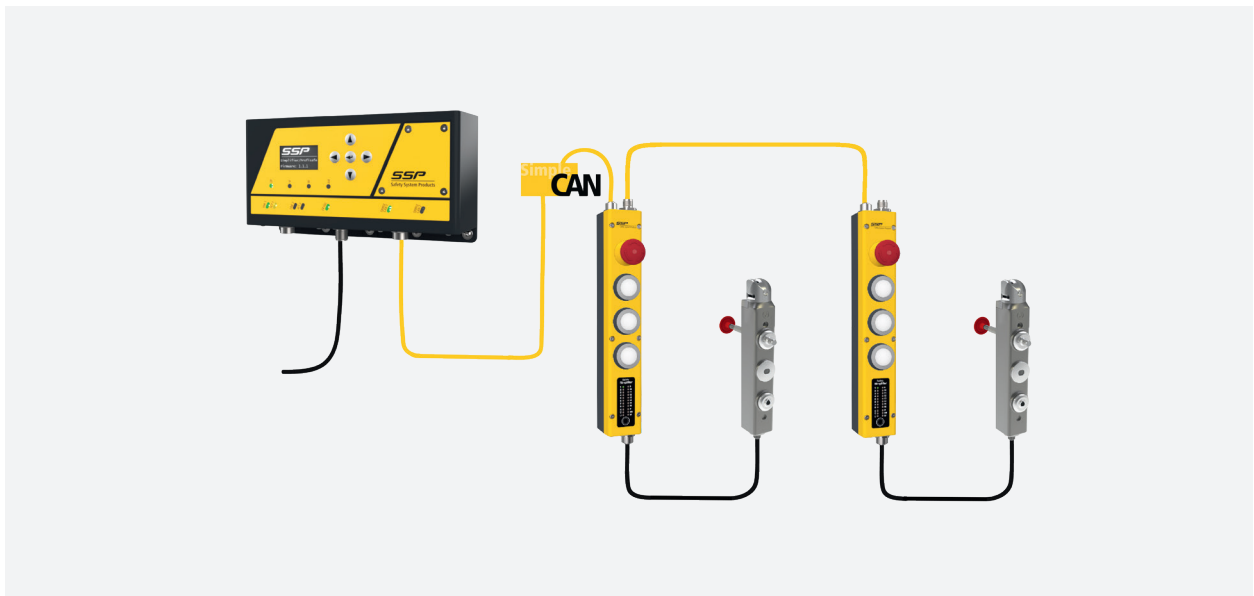
*Darstellung CAN-Vernetzung
