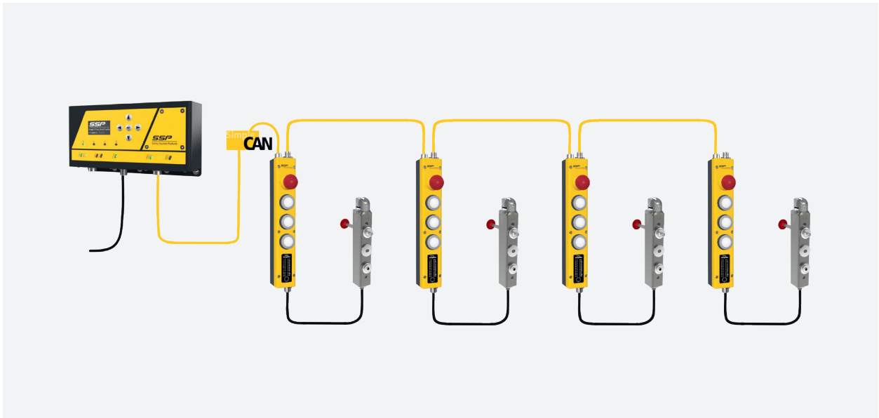
*Darstellung CAN-Vernetzung
