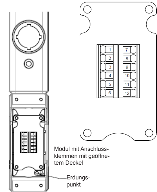
Selbstkonfektion - 12 Klemmen - TW1
