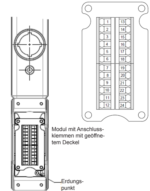
Selbstkonfektion - 24 Klemmen - TW3 & TW4
